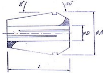
TOOL SUPPORT TYPE ER COLLET
